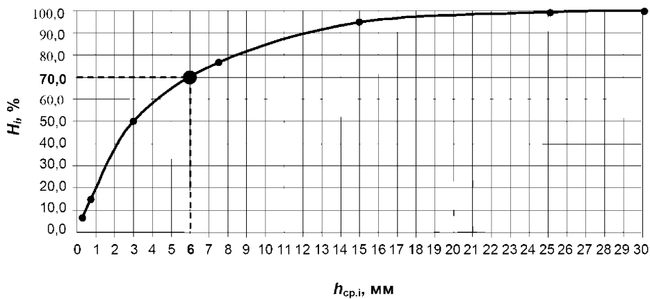
Рисунок И.1 Зависимость принимаемого на очистку суммарного за год слоя жидких осадков (%) от величины максимального суточного слоя дождя (мм), принимаемого на очистку в полном объеме, для г. Санкт-Петербург (по метеостанции Ленинград, ИЦП)
