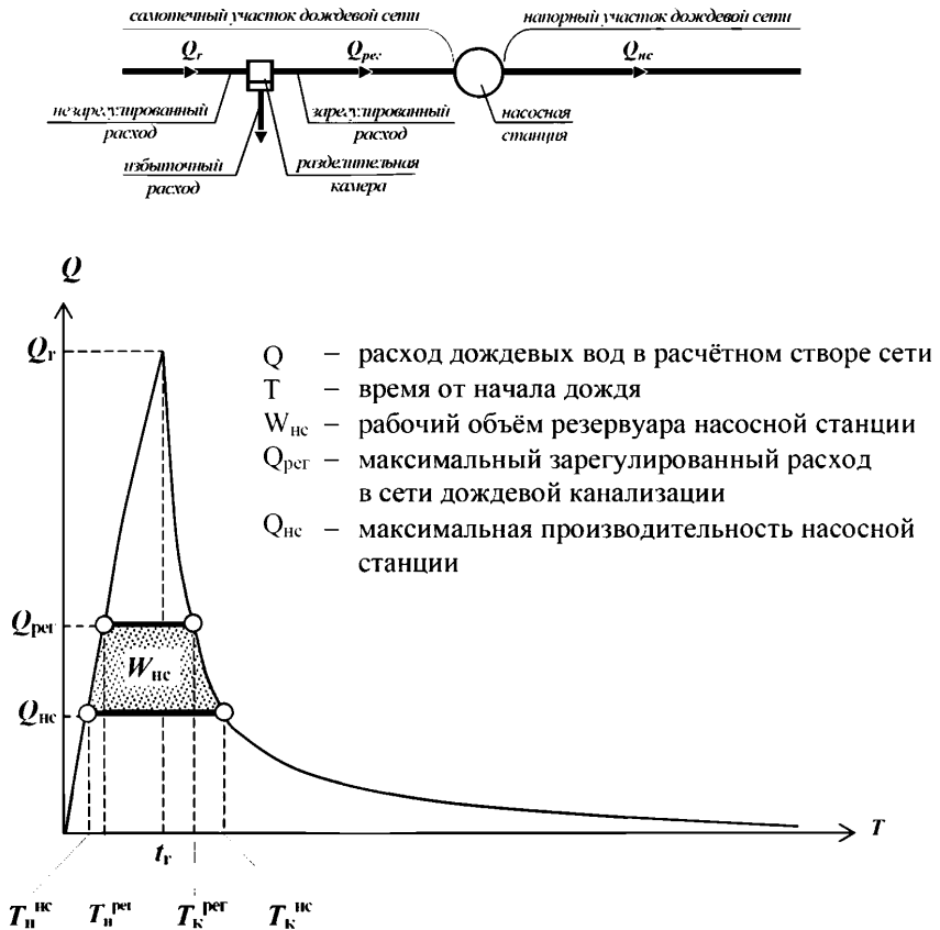
Рисунок Ж.2 Схема и расчётный гидрограф перекачки зарегулированного стока
