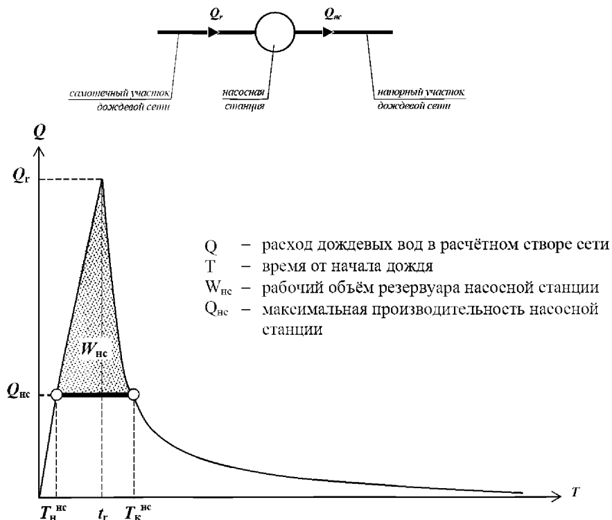
Рисунок Ж.1 Схема и расчётный гидрограф перекачки незарегулированного стока
