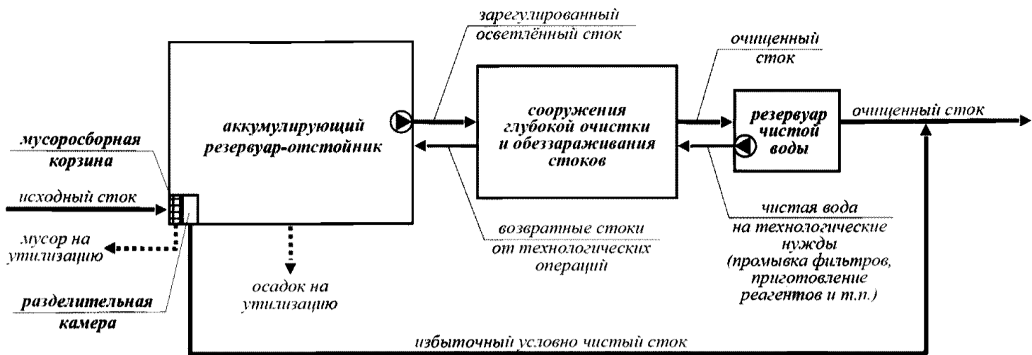
Схема 1 - с предварительным осветлением стока в аккумулярующем резервуаре
