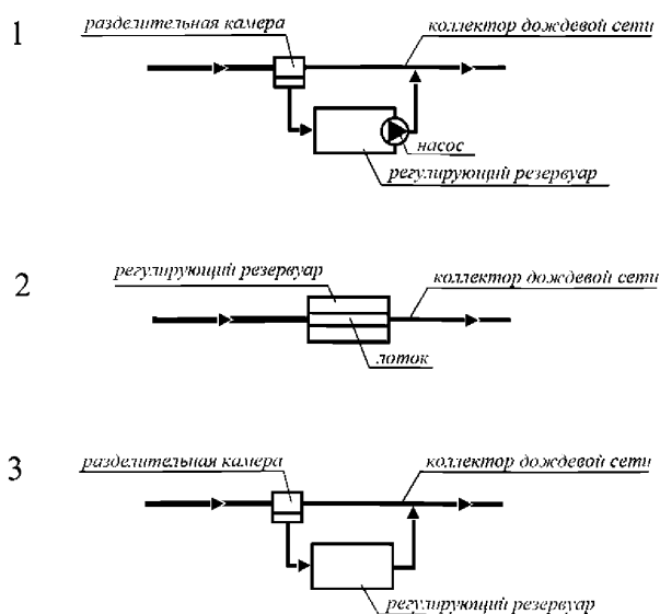
Рисунок 2. Принципиальные схемы регулирования расхода дождевого стока в сети дождевой канализации
