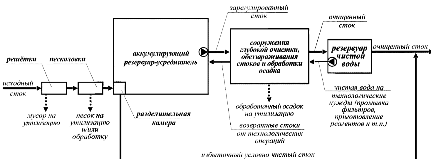
Схема 3 - с осаждением тяжёлых механических примесей (песка) перед разделением и аккумулярованием стока
