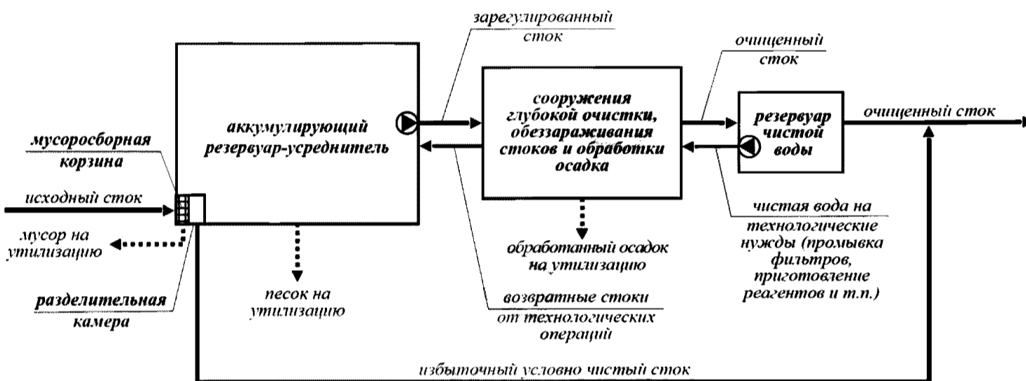
Схема 2 - с осаждением тяжёлых механических примесей (песка) в аккумулярующем резервуаре
