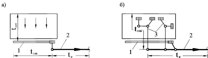
Рисунок 1 Схемы к определению продолжительности протекания дождевых вод t_r
